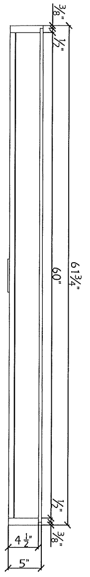
Section A-A
